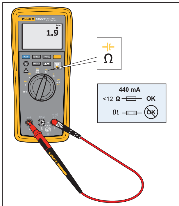
Figura 9. Prueba de los fusibles
