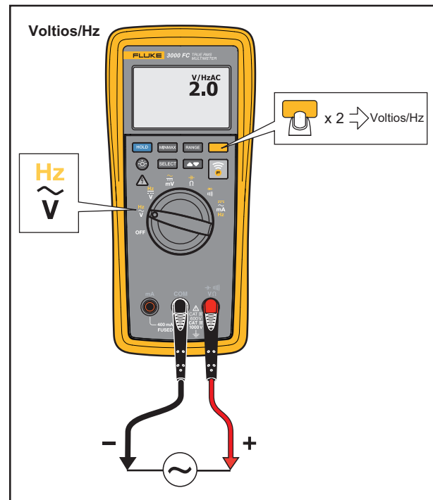
Figura 2. Relación de voltios/hercios
